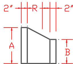
ER ECCENTRIC REDUCER
